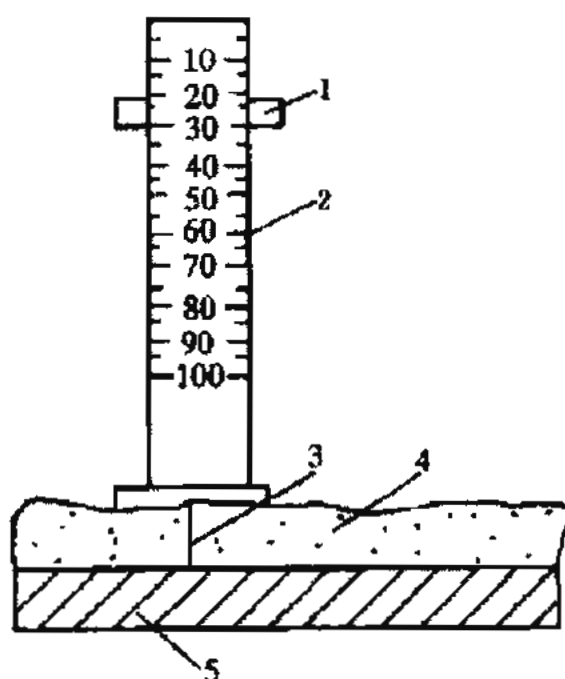
图 F.0.1 测厚度示意图
