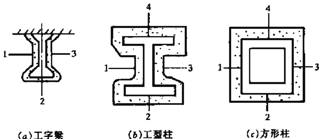
图 F.0.2 测点示意图
