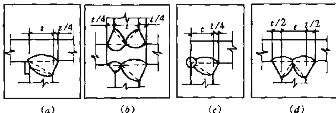
图 5.2.5 焊脚尺寸
