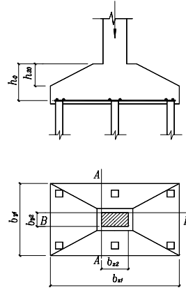
5.9.10-3 锥形承台斜截面受剪计算示意
