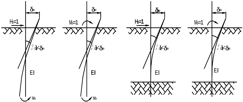
(a) 桩端支承在非岩石类土中或基岩表面 (b) 桩端嵌固于基岩中
