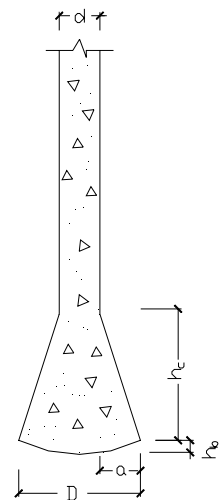
图 4.1.3 扩底桩构造
