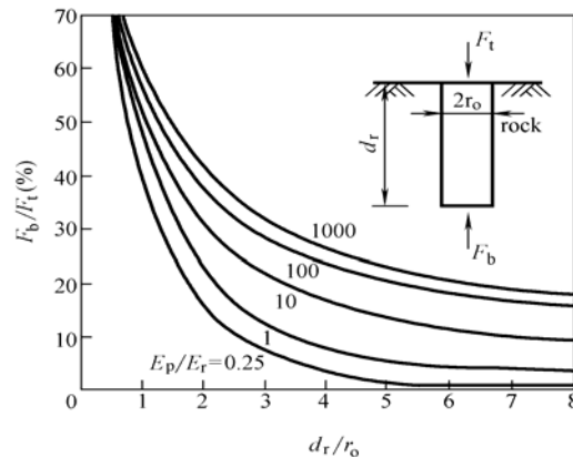
图 5.3-8 嵌岩桩端阻分担荷载比随桩岩刚度比和嵌岩深径比的变化 (引自 Pells and Turner, 1979)
