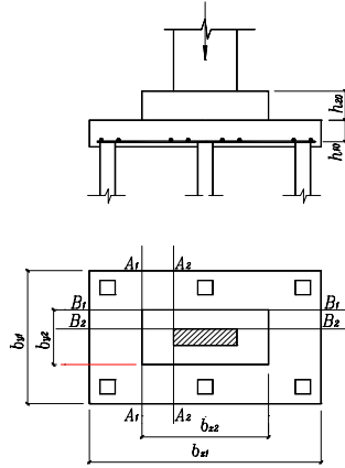
图 5.9.10-2 阶梯形承台斜截面受剪计算示意
