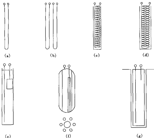
图3 竖直地埋管换热器形式
