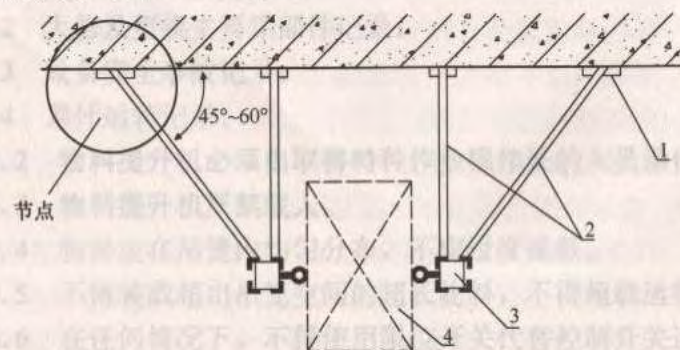
图 A.0.1-1 型钢附墙架与埋件连接
